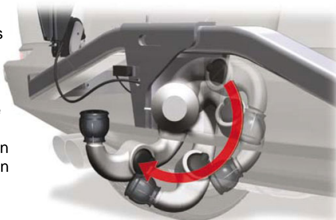
Abb.: Bosal Oris – Technologieführer bei den schwenkbaren AHVs
